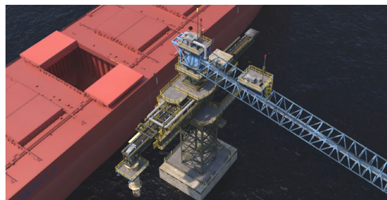
LaseCAU-ML ist ein fortschrittliches, sensorbasiertes Sicherheitssystem, das Kollisionen zwischen vertikalen Kranbalken, Schiffsluken und Rutschen verhindert.
